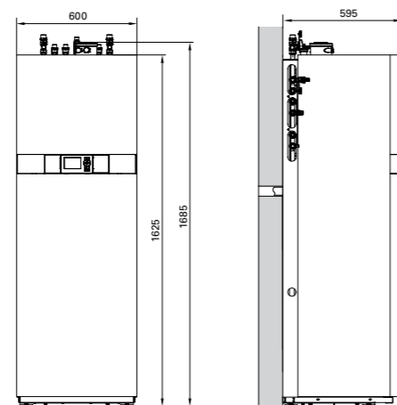
Vitodens 333-F, Type FR3A
