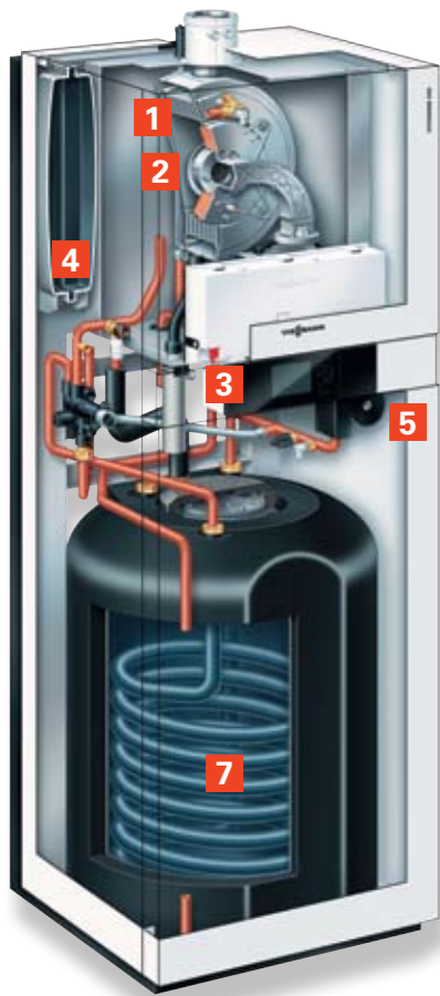
Vitodens 333-F met geëmailleerde spiraal-warmwaterboiler voor gebieden met hard water
