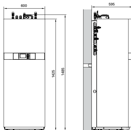
Vitodens 333-F, Type FS3A
