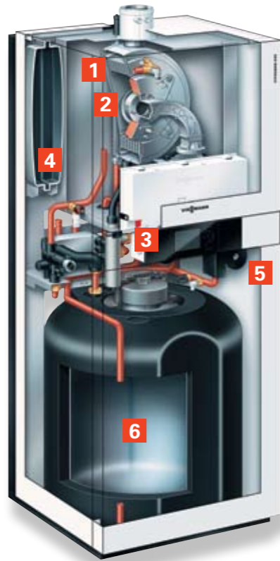
Vitodens 333-F met roestvast stalen laadboiler
